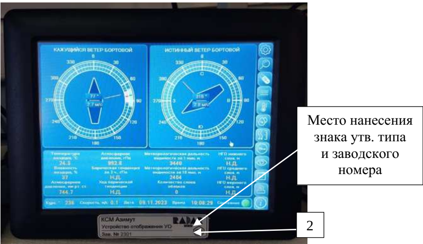
2- заводской номер Рисунок 3 – Общий вид устройство отображения УО комплексов Азимут и места нанесения заводского номера и знака утверждения типа
