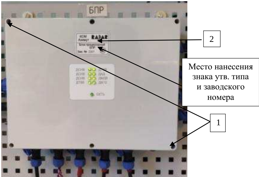
1- пломбировка, 2 – заводской номер Рисунок 2 – Общий вид блока БПР комплексов Азимут и места нанесения заводского номера и знака утверждения типа
